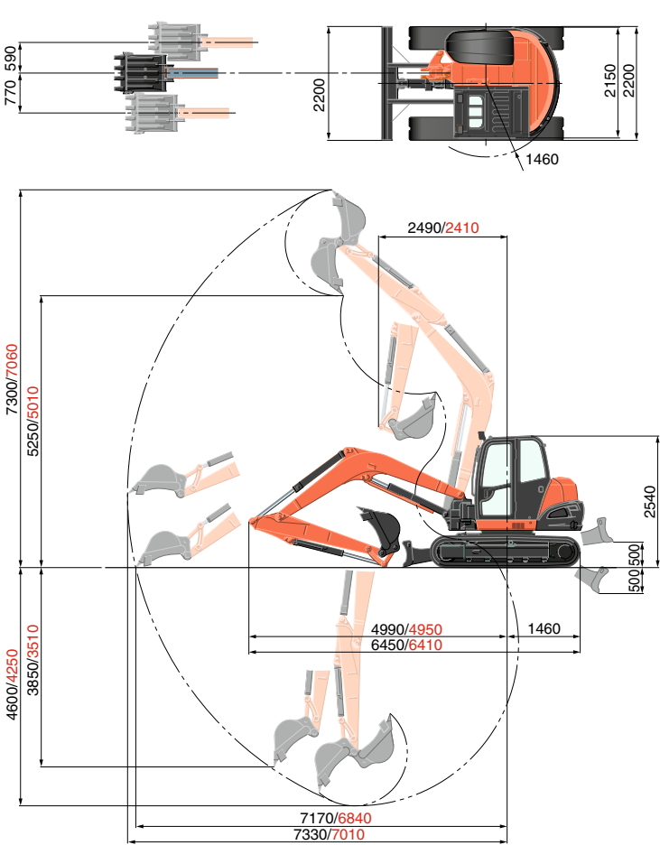
Balancier de 2100 mm Balancier de 1750 mm Unité:mm
